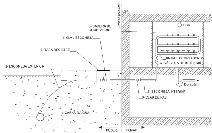
DETALL INSTAL·LACIÓ AMB SOTERRANI
