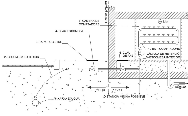
DETALL INSTAL·LACIÓ SENSE SOTERRANI
