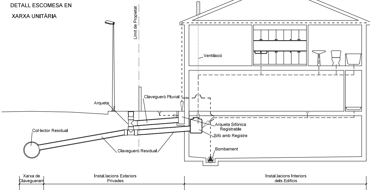
DETALL ORIENTATIU SIFÓ AMB REGISTRE
