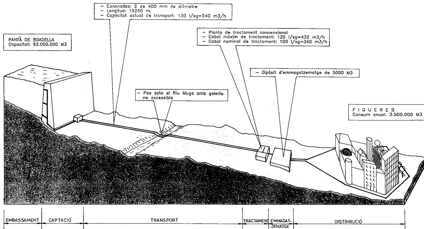
Perfil de captació, transport, tractament i distribució de l'aigua de Figueres.
